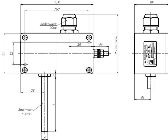
ТС (ТС.К, ТС.П) с головкой типа «Г8/2» (материал головки - алюминиевый сплав)
