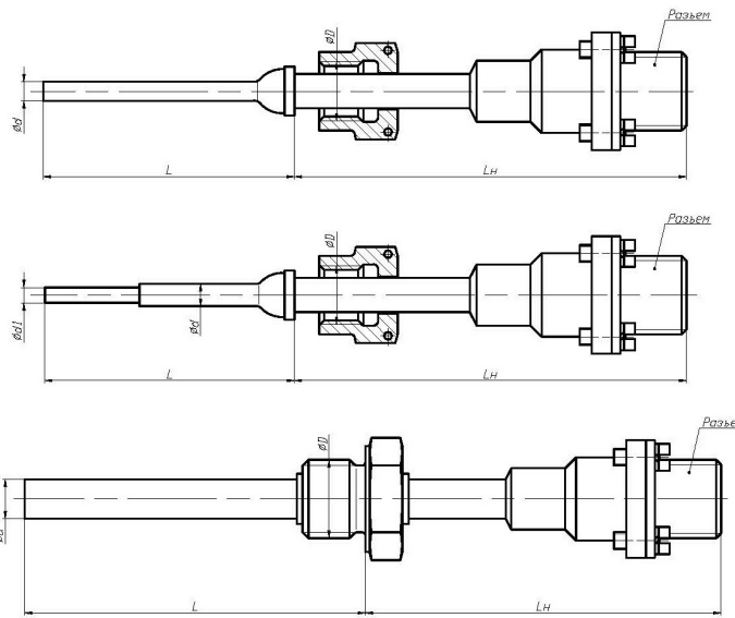
Рисунок Г.6 - Общий вид ТС без головки модели TCM 012 с разъемами типов 2PMГ, 2PMT
