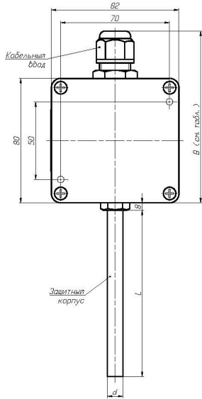
ТС (ТС.К, ТС.П) с головкой типа «Г9» (материал головки - поликарбонат)
