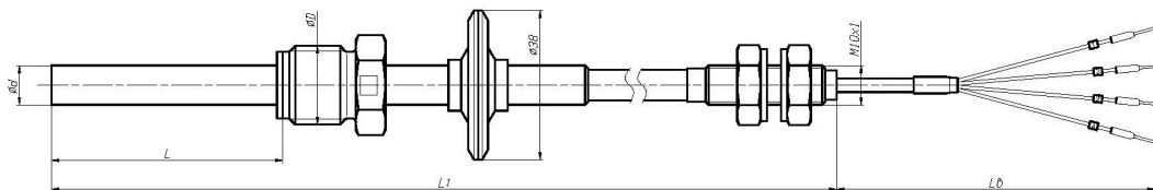
Рисунок Г.8 - Общий вид ТС без головки модели TCM(TCP) 012.15
