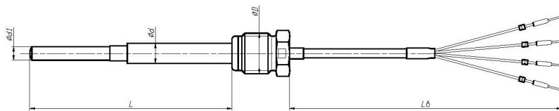
Рисунок Г.7 - Общий вид ТС без головки модели TCM(TCP) 012.12
